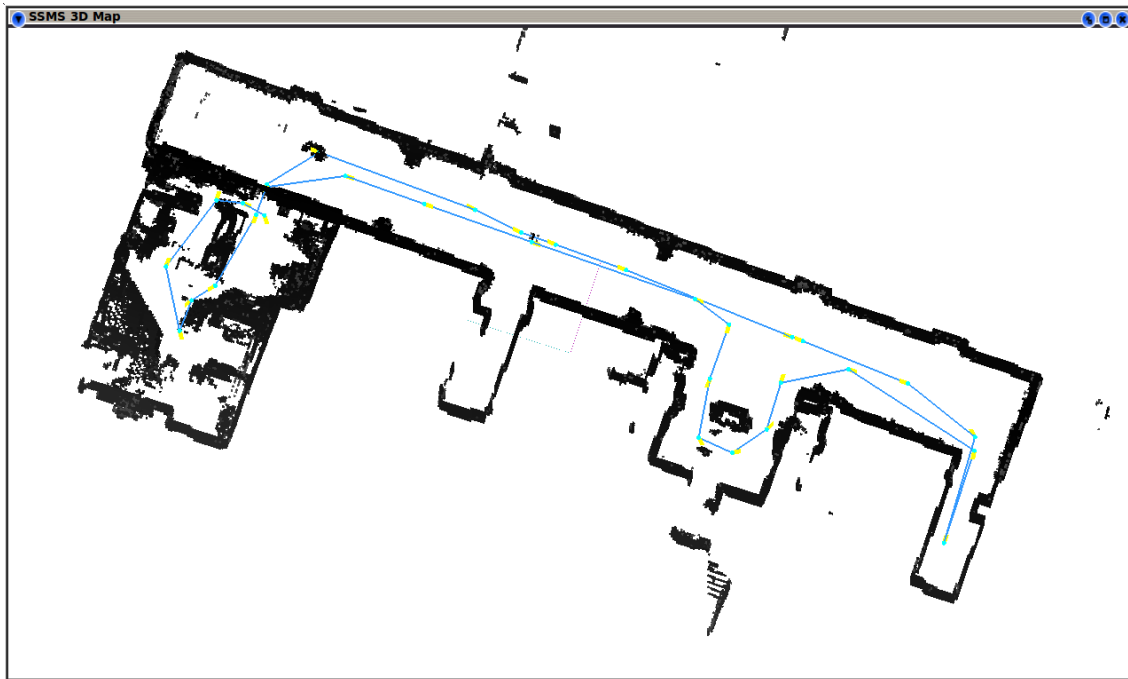
Figura 5.11: Vista aérea oblicua del mapa de superficies multinivel conjunto para el pasillo y el laboratorio tras ser corregidas las posiciones por el algoritmo SLAM 6D. La línea marca la trayectoria seguida por el robot y los puntos la posición desde la que se tomó el scan
